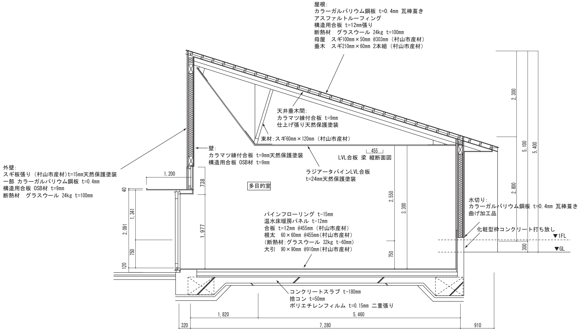
企画展示室断面図 縮尺 1/120
